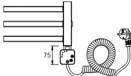
EGUUS.ERHT2C regulátor povrchové teploty se sí ovou vidlicí
